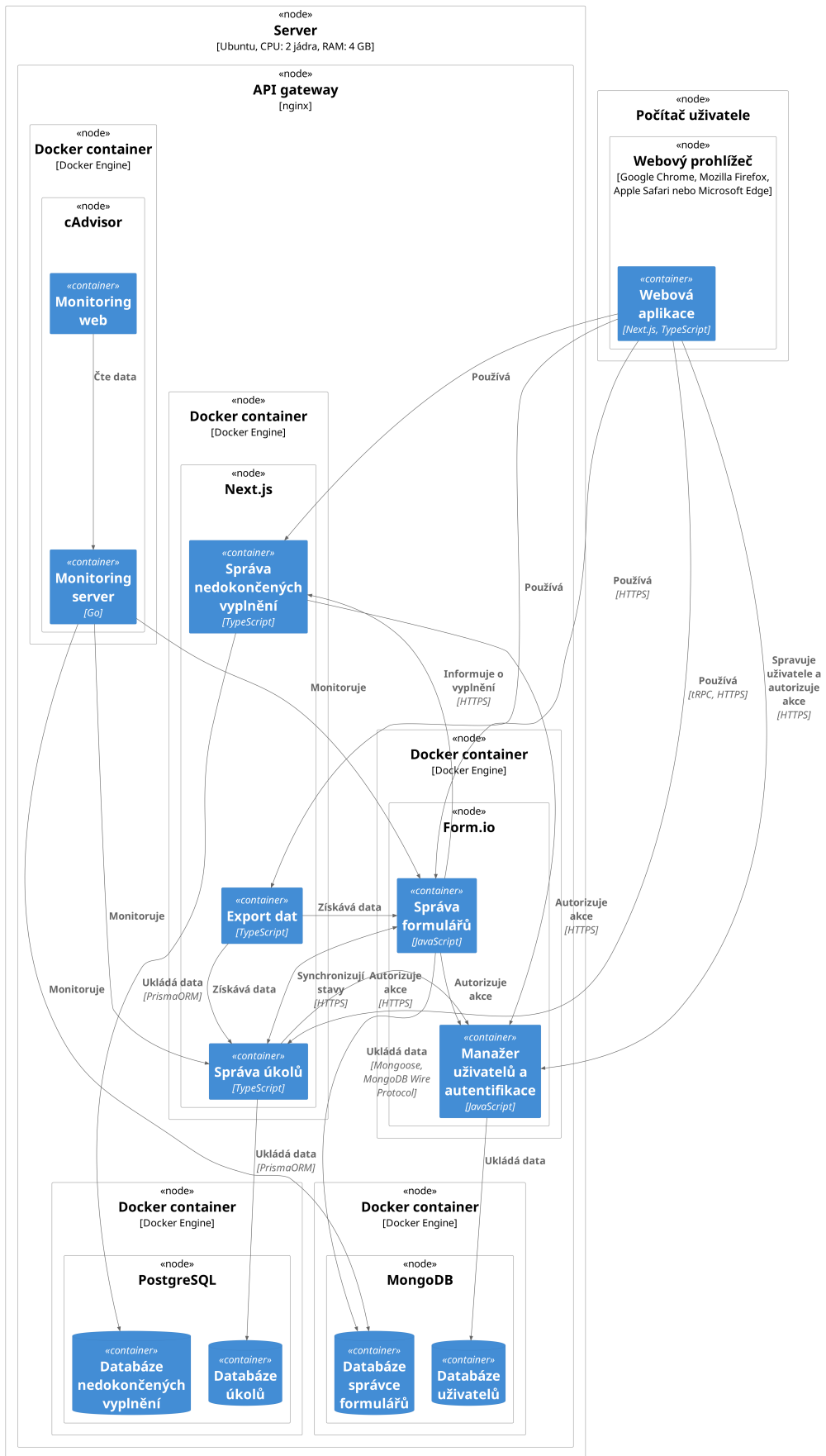
Obrázek 3.4: Diagram nasazení
